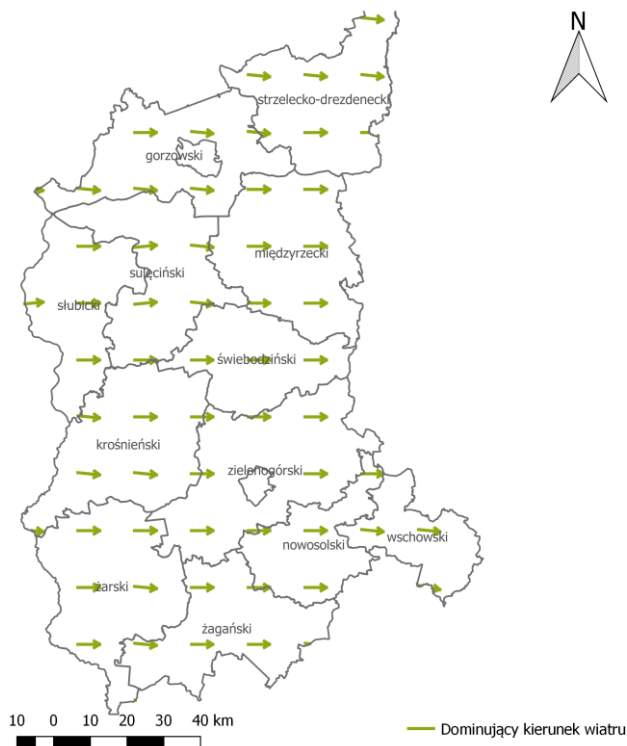
Rysunek 1-8 Dominujący w roku kierunek wiatru wyznaczony na przez model WRF/CALMET dla strefy lubuskiej w 2016 r.
