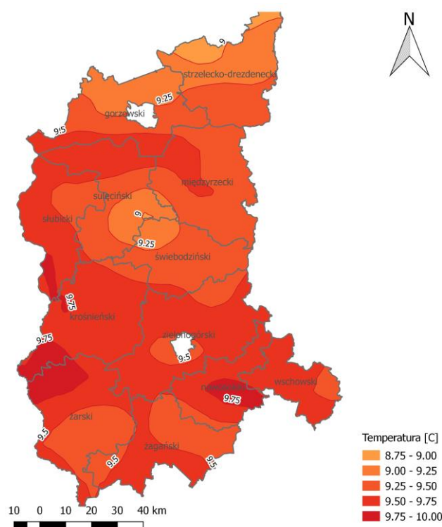
Rysunek 1-13 Przestrzenny rozkład średnich rocznych wartości temperatury powietrza wyznaczonych przez WRF/CALMET w strefie lubuskiej w 2016 r.
