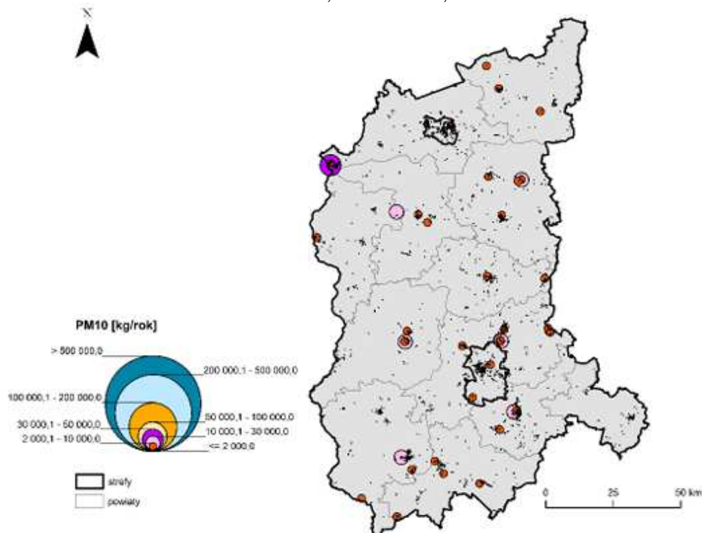
Rysunek 17. Lokalizacja punktowych źródeł emisji PM 10 na obszarze województwa lubuskiego w 2021 roku.
