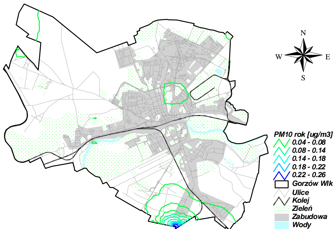
Rysunek 37 Stężenia PM_{10} rok w Gorzowie Wielkopolskim pochodzące od emitorów punktowych zlokalizowanych w pasie 30km od miasta w 2005r.
