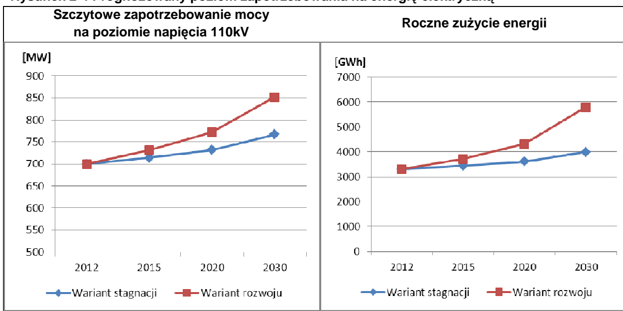
Rysunek 2-4 Prognozowany poziom zapotrzebowania na energię elektryczną
