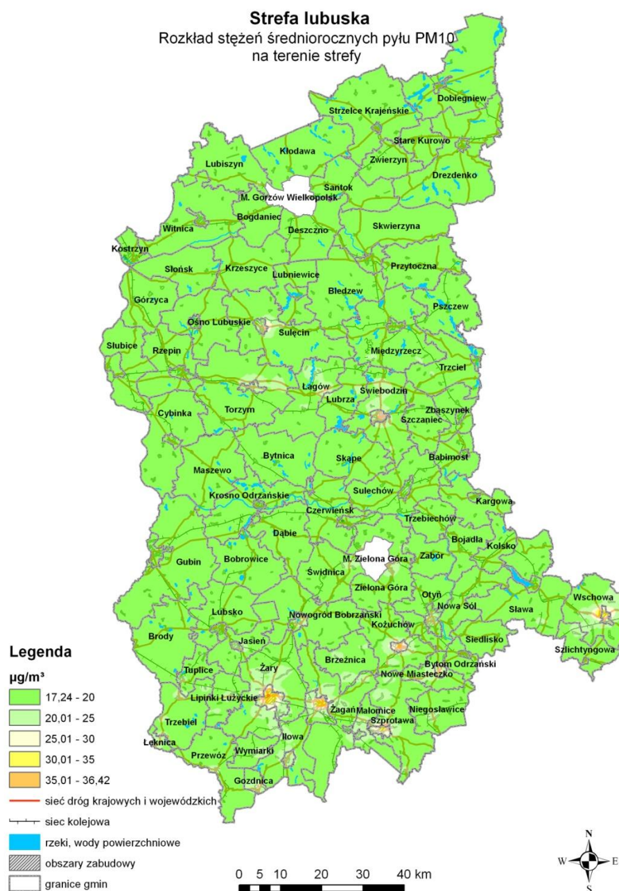
Rysunek 18. Rozkład stężeń średniorocznych pyłu zawieszonego PM10 w strefie lubuskiej w roku bazowym 2011 53
