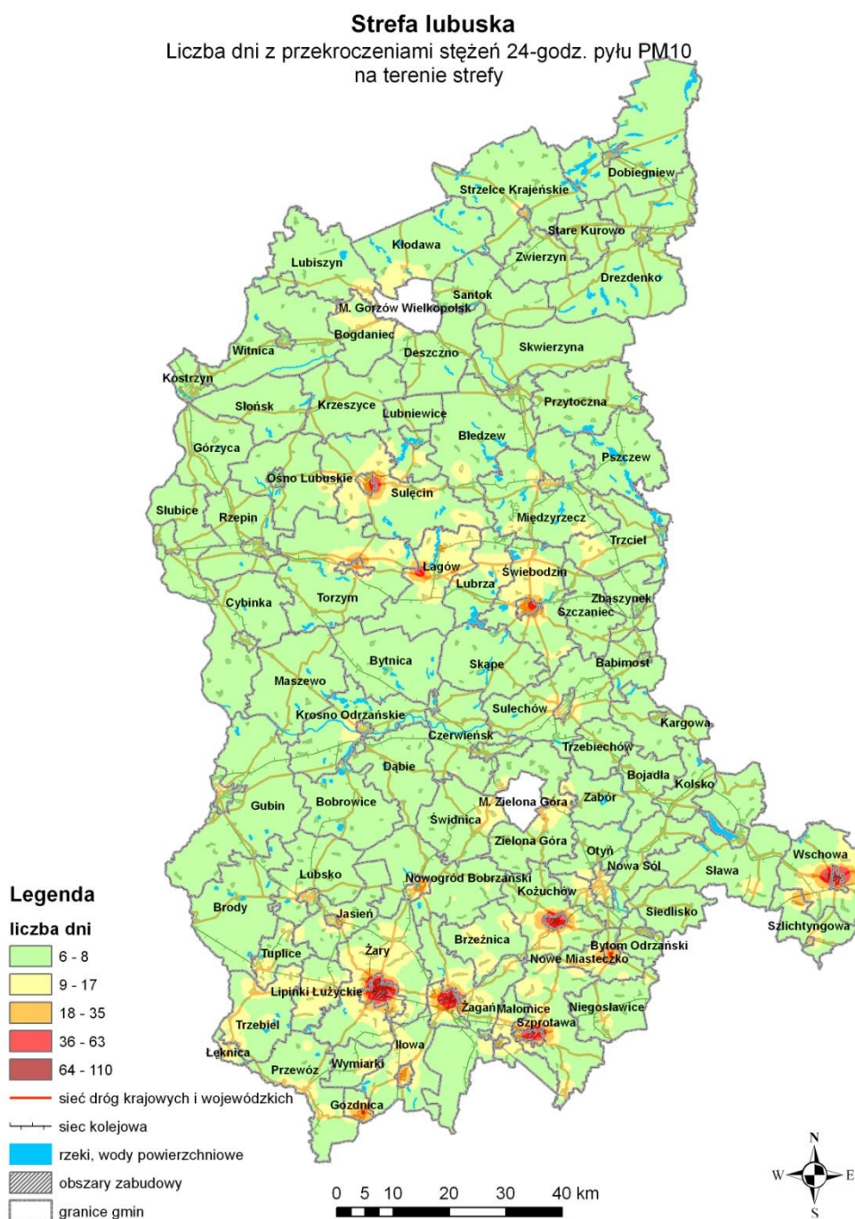
Rysunek 19. Rozkład liczby dni z przekroczeniem dopuszczalnej wartości stężenia 24-godzinne dla pyłu zawieszony PM10 w strefie lubuskiej w roku bazowym 2011 54
