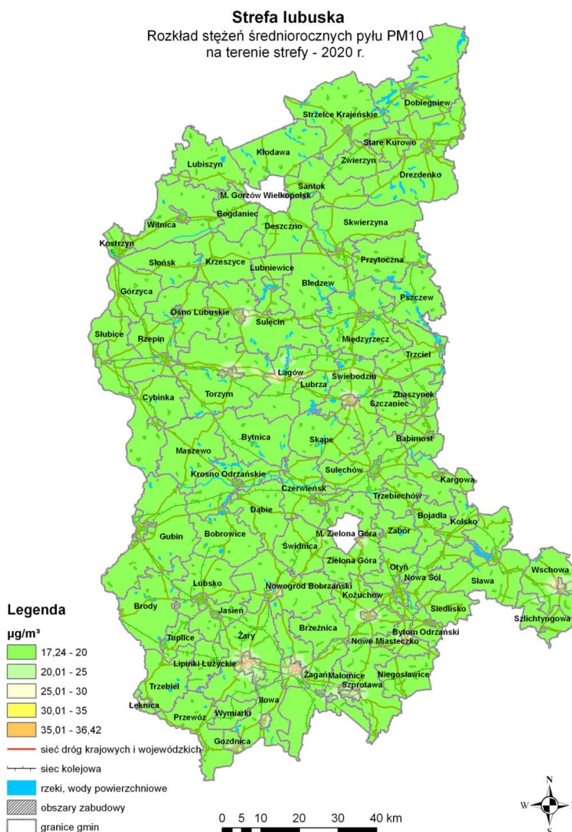
Rysunek 34 Rozkład stężeń średniorocznych pyłu PM10 na obszarze strefy lubuskiej w roku prognozy 2020 79 .
