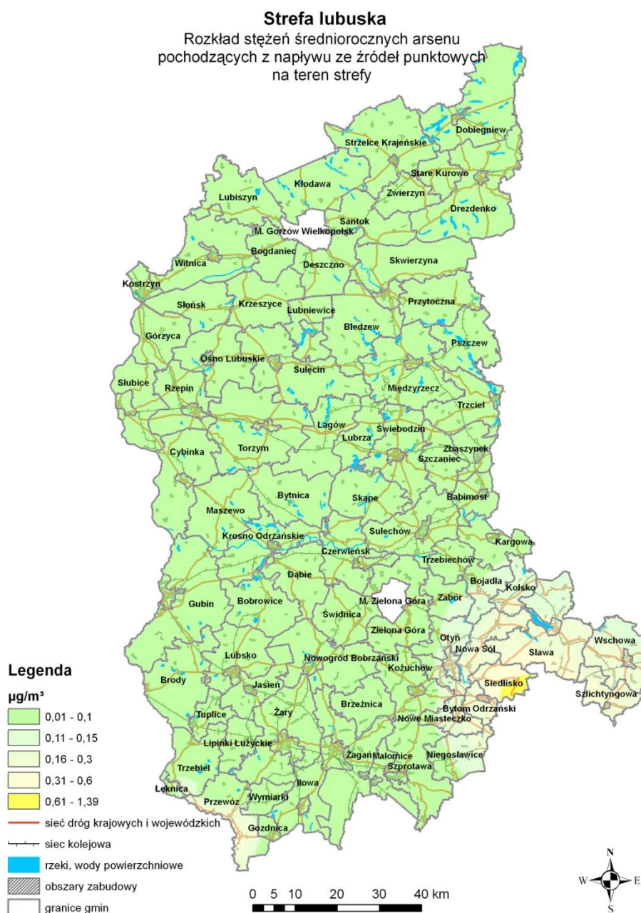
Rysunek 22. Rozkład stężeń średniorocznych arsenu w strefie lubuskiej w roku bazowym 2011 57
