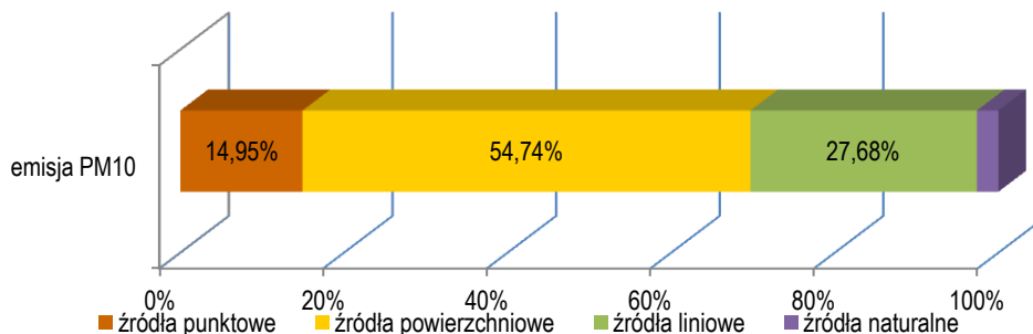
Rysunek 29. Procentowe udziały poszczególnych źródeł emisji, w rocznej emisji pyłu zawieszonego PM10, w strefie lubuskiej
