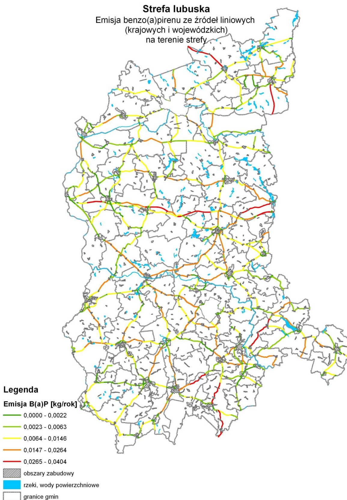
Rysunek 46. Rozkład emisji benzo(a)pirenu z dróg krajowych i wojewódzkich w strefie lubuskiej
