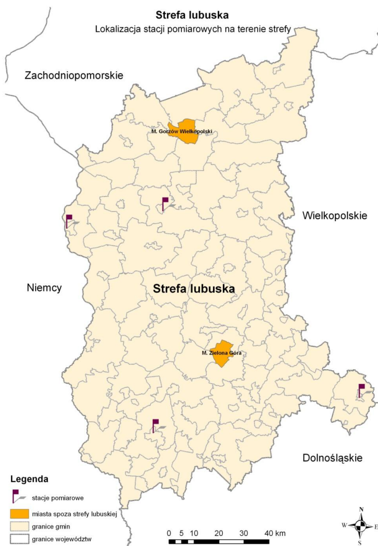
Rysunek 2 Lokalizacja stacji pomiarowych w strefie lubuskiej w 2011 roku 21
