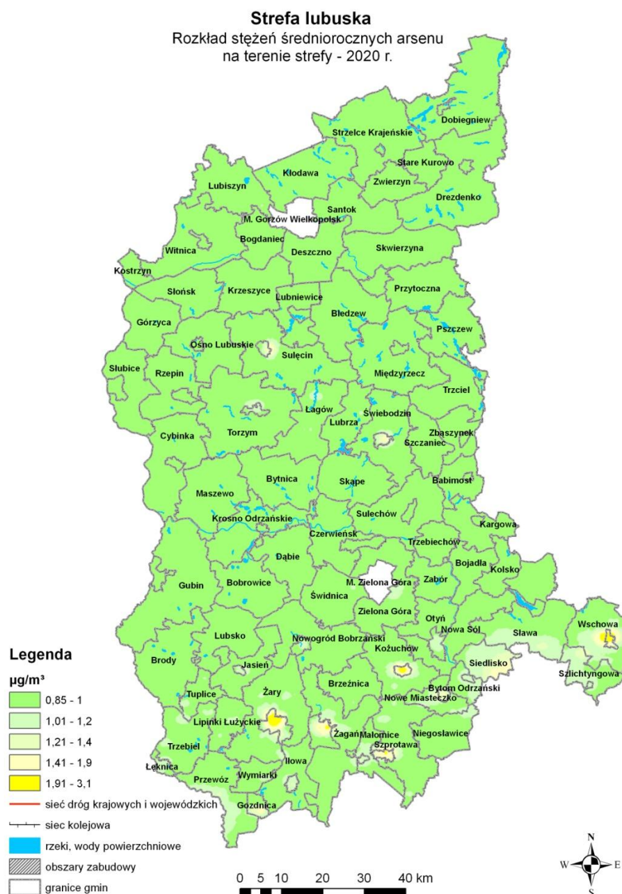
Rysunek 37 Rozkład stężeń średniorocznych arsenu na obszarze strefy lubuskiej w roku prognozy 2020
