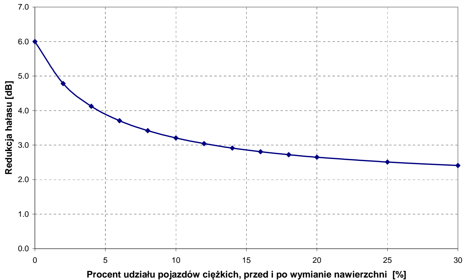
Rys. 8. Redukcja hałasu samochodowego na skutek wymiany nawierzchni drogi na cichą
