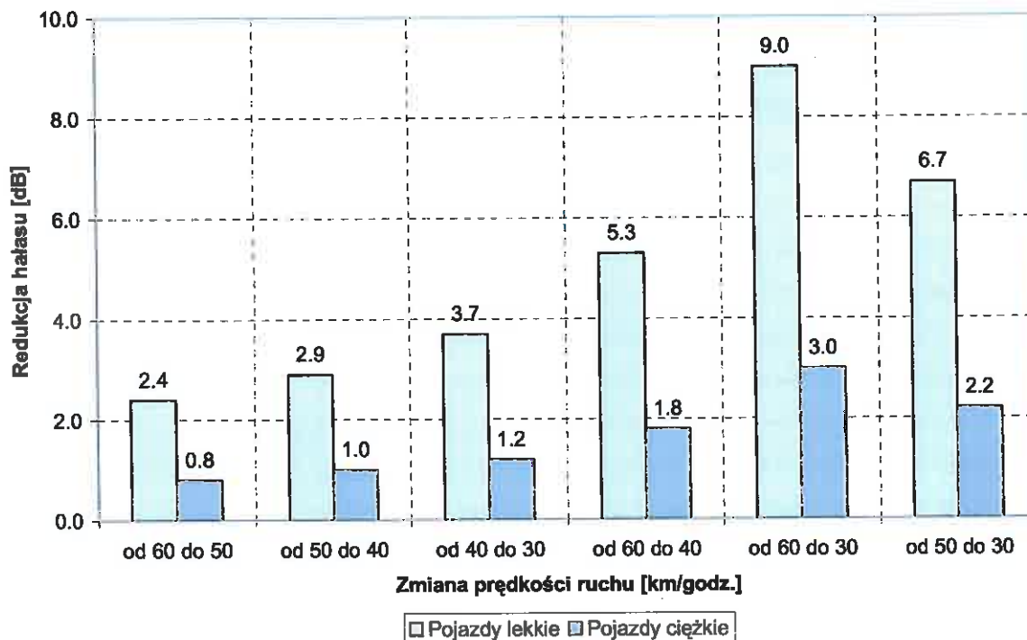
Rys. 31. Redukcja hałasu pojazdów lekkich i ciężkich, w zależności od zmiany prędkości ruchu
