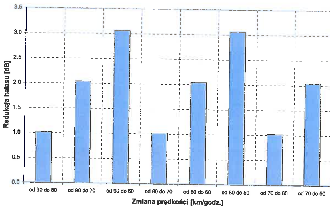
Rys. 30. Redukcja hałasu pojazdów ciężkich, w zależności od zmiany prędkości ruchu
