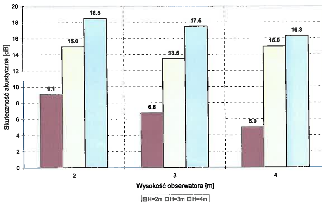
Rys. 39. Skuteczność akustyczna ekranu (odległość ekranu od źródła dźwięku: 4.0 m, odległość punktu obserwacji od ekranu: 10.0 m)
