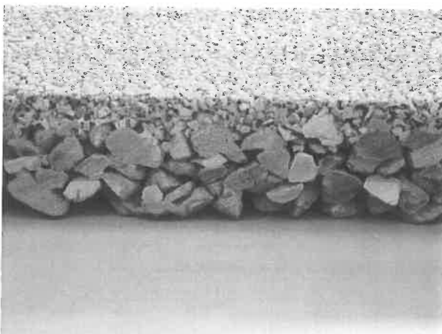
Rys. 36. Budowa nawierzchni dwuwarstwowej
