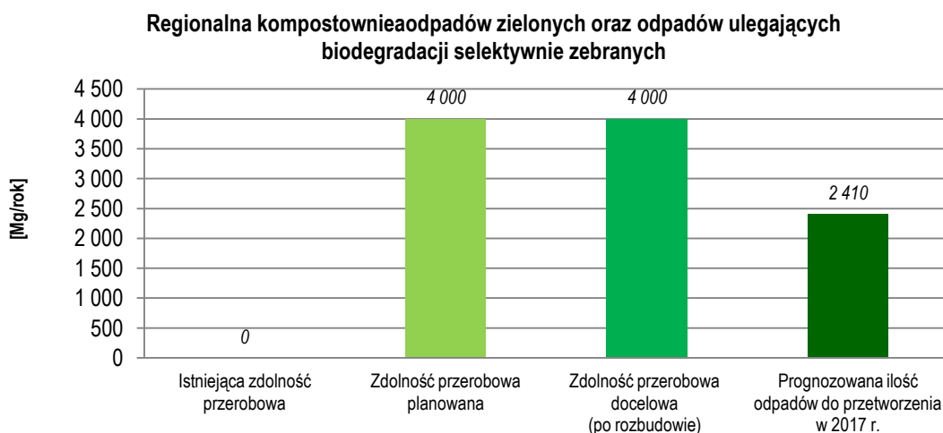
Rysunek 26. Bilans masowy istniejącej oraz planowanej regionalnej instalacji do przetwarzania selektywnie zebranych odpadów zielonych i innych odpadów ulegających biodegradacji (kompostowni) w stosunku do prognozowanych ilości wytworzonych odpadów w 2017 r., przeznaczonych do kompostowania
