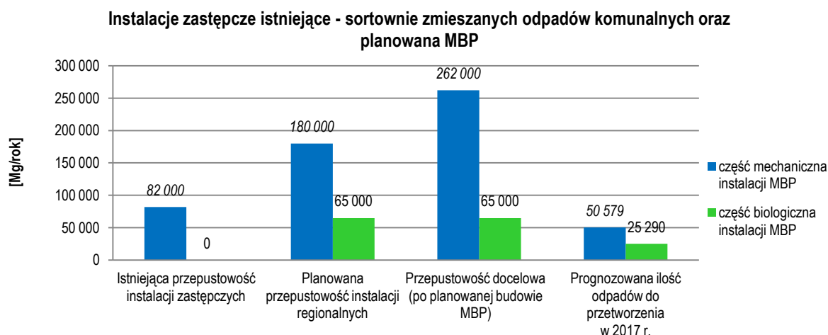
Rysunek 13. Bilans masowy istniejących instalacji zastępczych oraz planowanych instalacji MBP w stosunku do ilości odpadów prognozowanych w 2017 r. – region centralny
