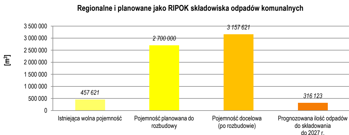
Rysunek 14. Bilans masowy istniejących regionalnych składowisk odpadów komunalnych w stosunku do ilości odpadów przeznaczonych do składowania do 2027 r. – region centralny
