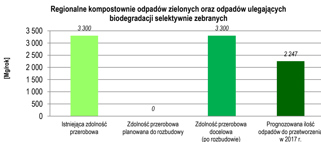
Rysunek 12. Bilans masowy istniejącej regionalnej kompostowni odpadów zielonych oraz odpadów ulegających biodegradacji selektywnie zebranych w stosunku do ilości odpadów prognozowanych w 2017 r. – region centralny
