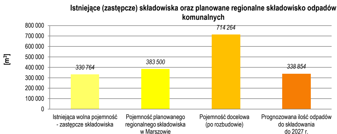
Rysunek 25. Bilans masowy istniejących (zastępczych) składowisk odpadów komunalnych oraz planowanego regionalnego składowiska odpadów komunalnych w stosunku do ilości odpadów przeznaczonych do przetworzenia w 2017 r. – region zachodni
