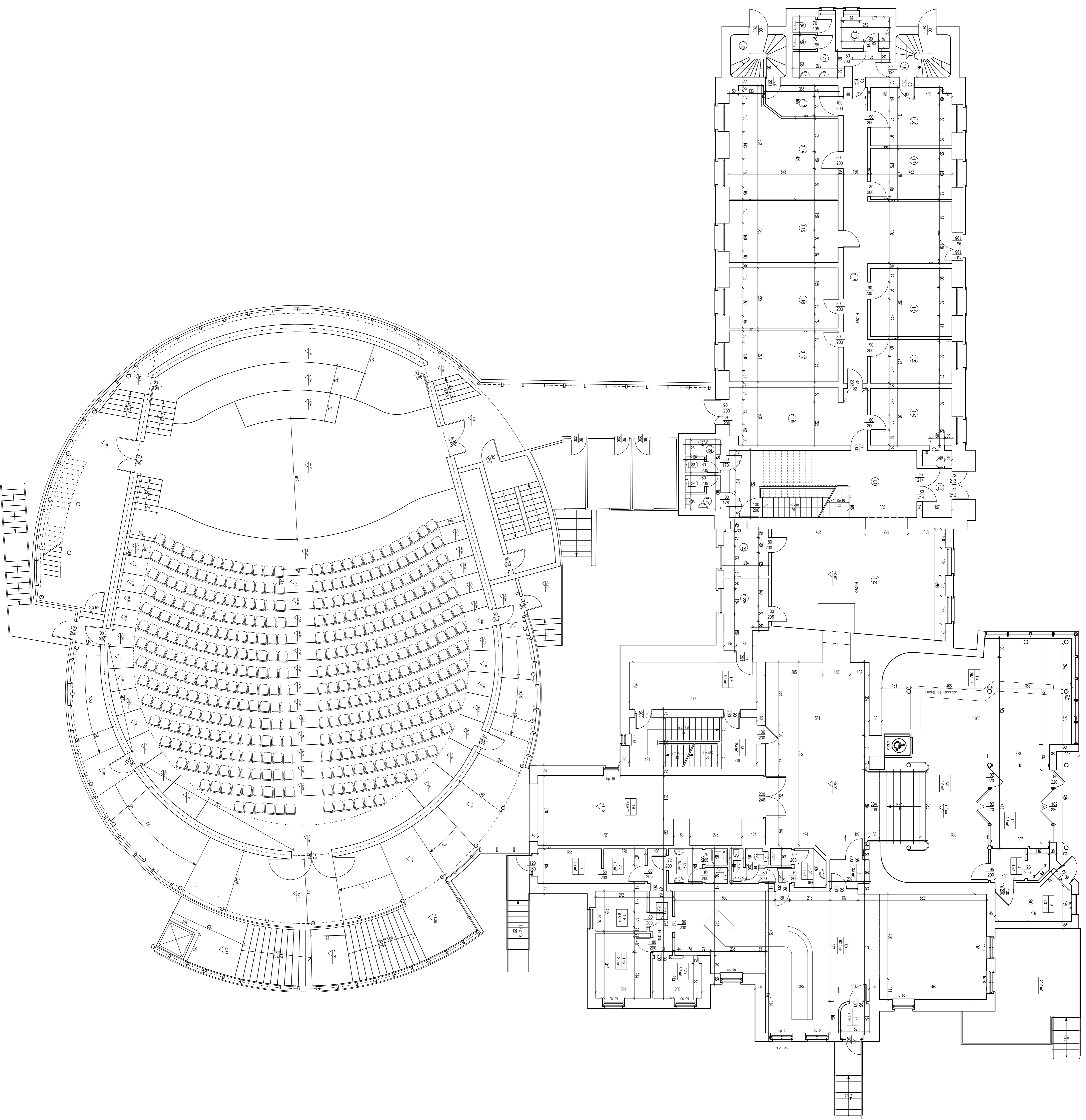
RZUT PRZYZIEMIA skala 1:100
