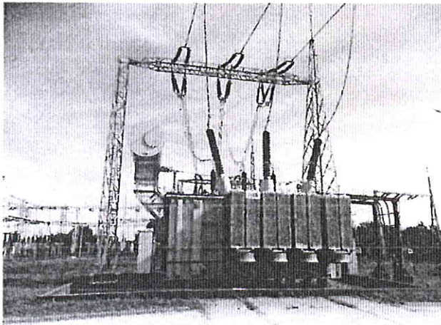
Autotransformator AT1 strona 220 kV
