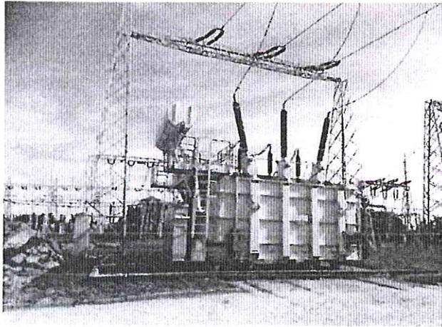
Autotransformator AT3 strona 220 kV
