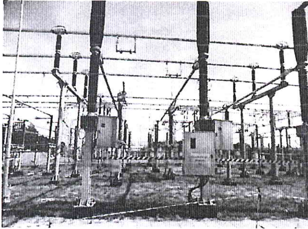
Pole 220 kV – Łącznik szyn
