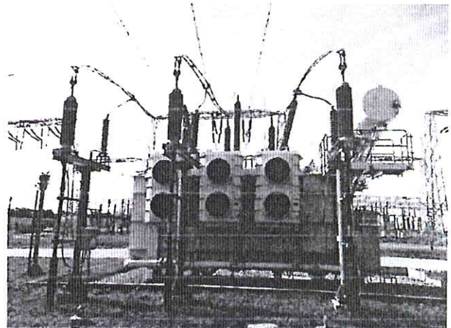
Autotransformator AT3 strona 110 kV
