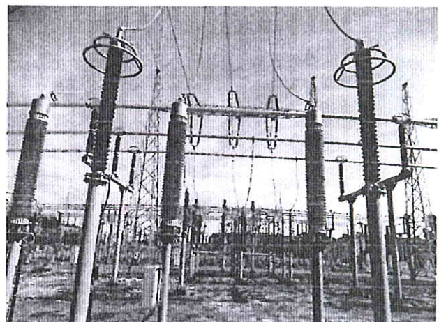
Pole 220 kV – linia Żukowice
