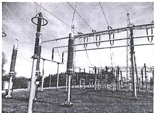
Pole 220 kV – linia Gorzów
