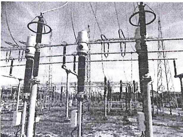
Pole 220 kV – linia Zielona Góra
