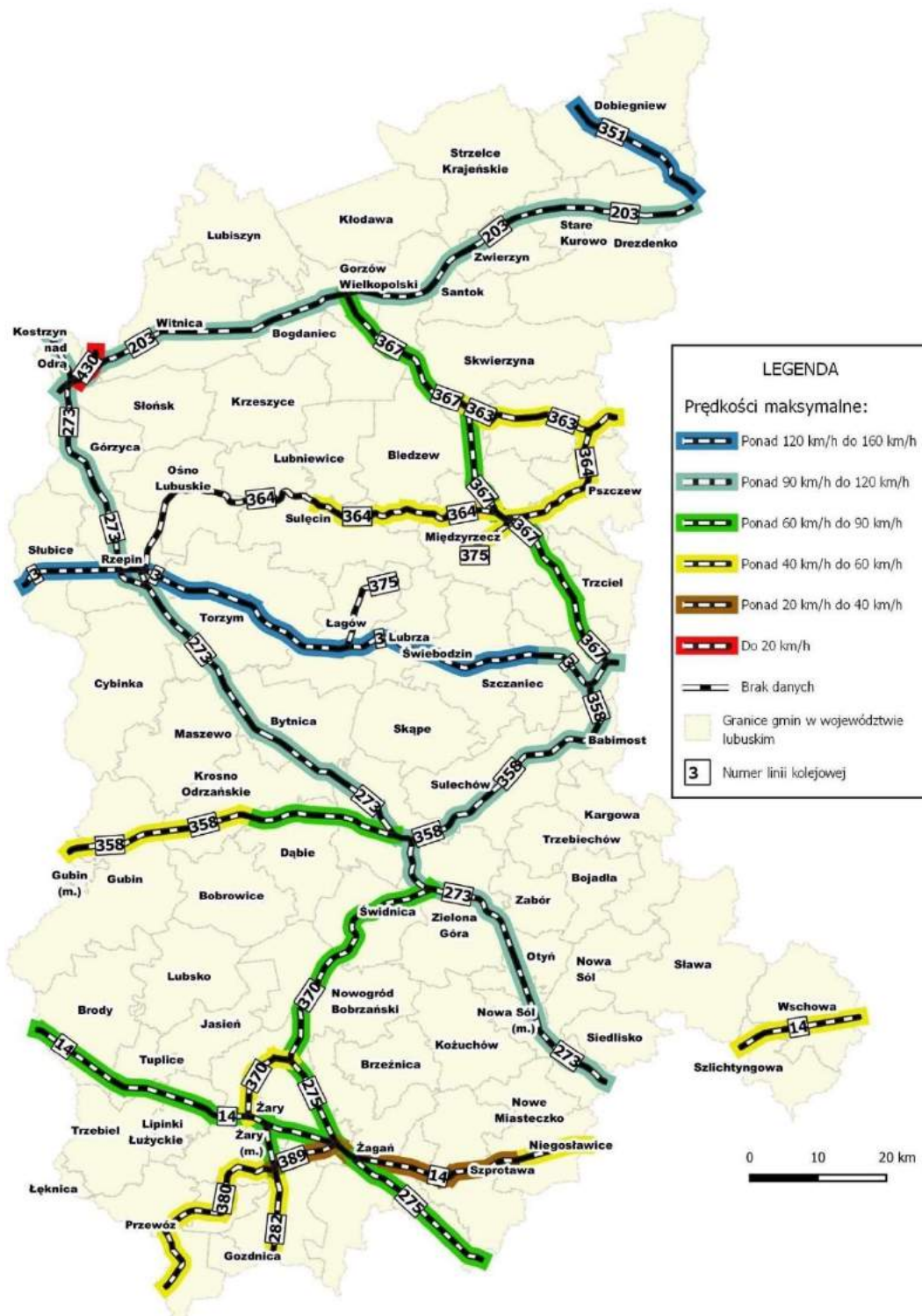
Rysunek 26. Prędkości maksymalne na sieci kolejowej
