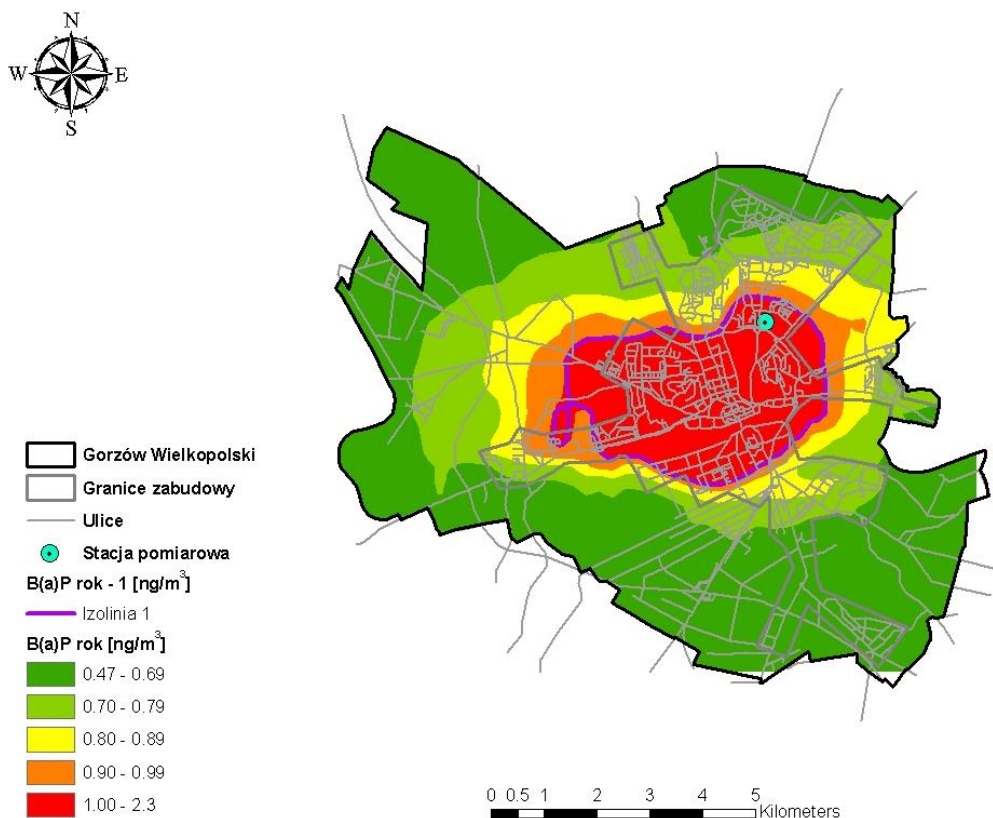
Rysunek 28 Stężenia B(a)P o okresie uśredniania wyników pomiarów rok kalendarzowy strefie miasto Gorzów Wielkopolski będące oddziaływaniem całkowitej emisji w 2010 r.
