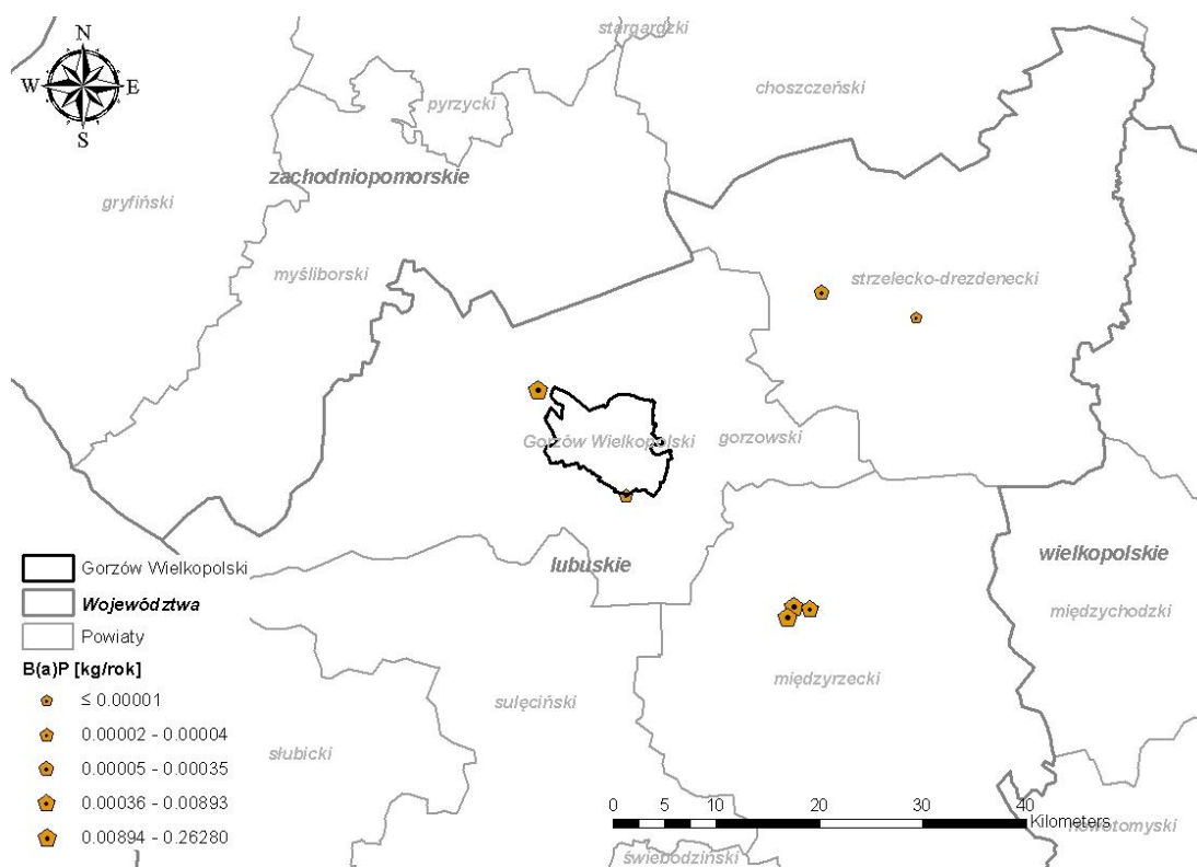
Rysunek 15 Lokalizacja instalacji, których eksploatacja powoduje wprowadzenie do powietrza B(a)P, rozmieszczonych w pasie 30 km wokół strefy miasto Gorzów Wielkopolski – emisja punktowa
