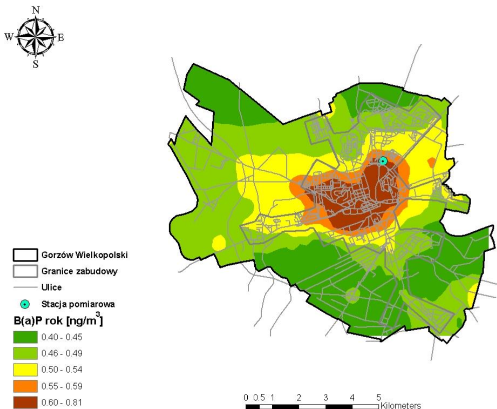
Rysunek 31 Stężenia B(a)P o okresie uśredniania wyników pomiarów rok kalendarzowy strefie miasto Gorzów Wielkopolski będące oddziaływaniem całkowitej emisji po zastosowaniu scenariusza – obniżenie emisji B(a)P o 80% z ogrzewania indywidualnego
