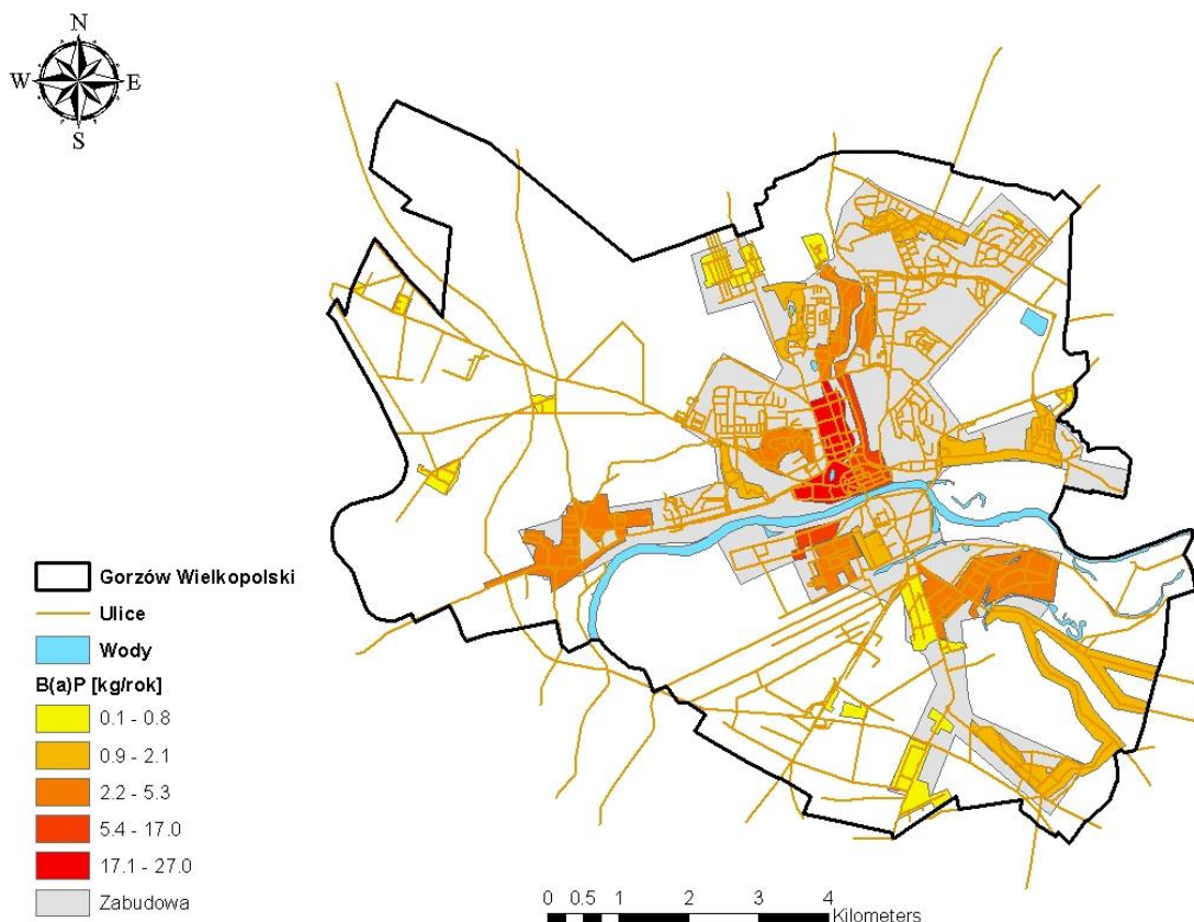
Rysunek 20 Lokalizacja instalacji, których eksploatacja powoduje wprowadzenie do powietrza B(a)P, rozmieszczonych na terenie strefy miasto Gorzów Wielkopolski – emisja powierzchniowa
